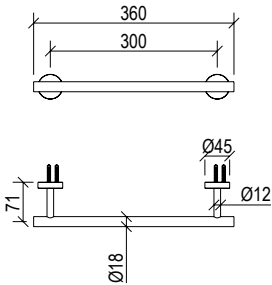
Porta salvietta lunga 300 mm in acciaio inox 316L.
