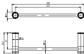
Porta salvietta lungo 300 mm in acciaio inox 316L.
