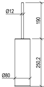
Porta scopino da appoggio in acciaio inox 316L.
