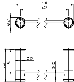
Porta salvietta lungo 450 mm in acciaio inox 316L.
