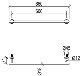
Porta salvietta lunga 600 mm in acciaio inox 316L.
